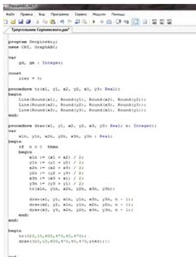
Рисунок 3. Готовая программа в PascalABC.NET
